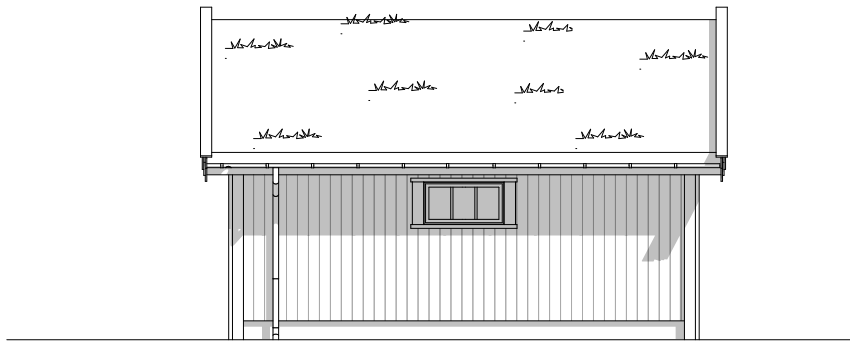
Fasade 1
